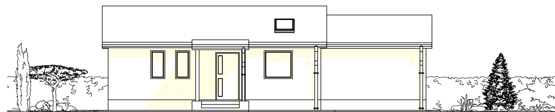
POHLED ZADNÍ
